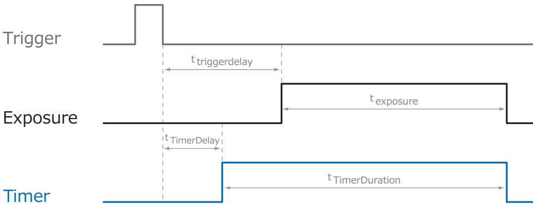
▼ 図40 BaumerMXGカメラでのタイマー設定
