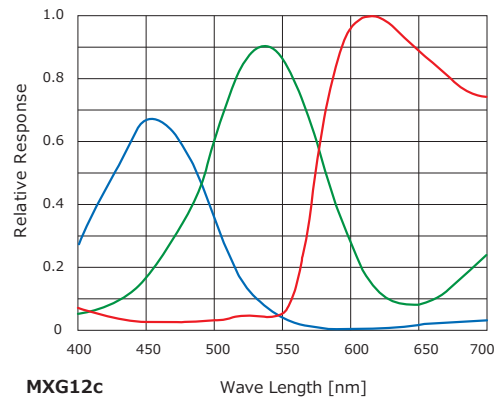
▼ 図7 1.2MP CCDセンサーを 搭載したBumaerMXG カメラの分光感度特性
