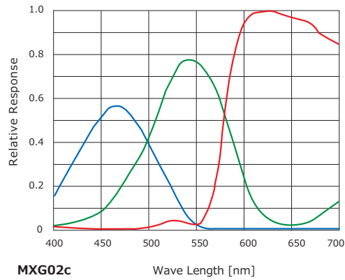
▼ 図6 0.3MP CCDセンサーを 搭載したBumaerMXG カメラの分光感度特性
