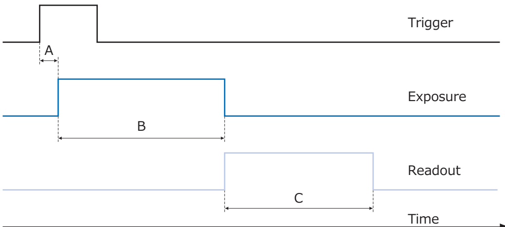
▲ 図36 Baumerカメラでの適切なトリガー信号
