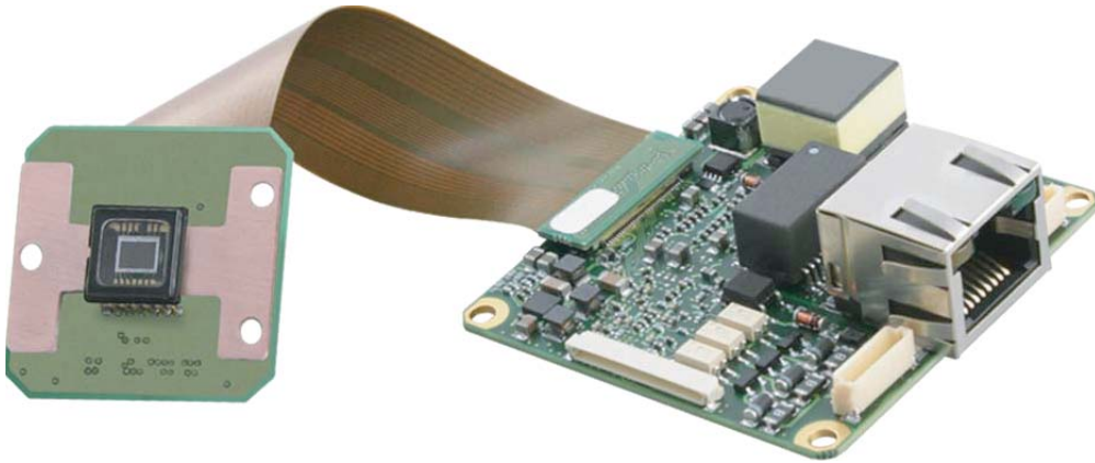
▼ 図1 Baumer MXGカメラの 画像
