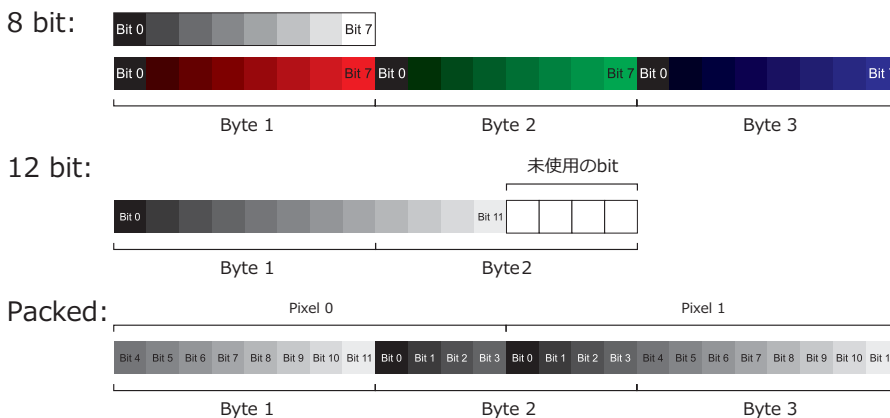
▼ 図14 モノクロ 8bitとRGB 8bitのデータ構成
