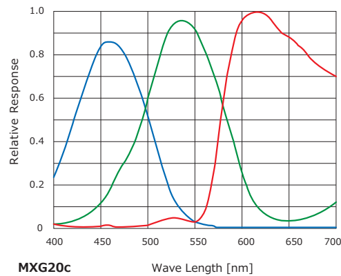
▼ 図8 2.0MP CCDセンサーを 搭載したBumaerMXG カメラの分光感度特性
