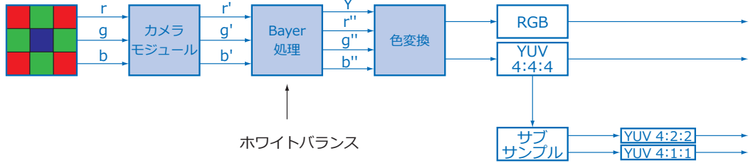
図29 ▼ Baumerカラーカメラの カラー化処理の工程
