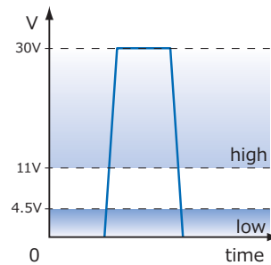
▲ 図36 Baumerカメラでの適切なトリガー信号
