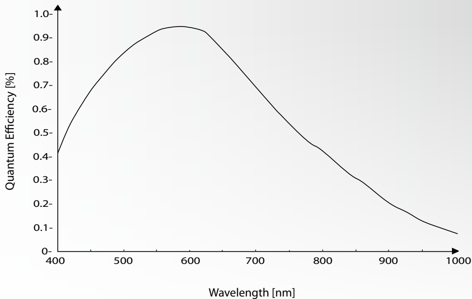
Sensor: Sony ICX 445ALA - courtesy of SONY Deutschland GmbH
