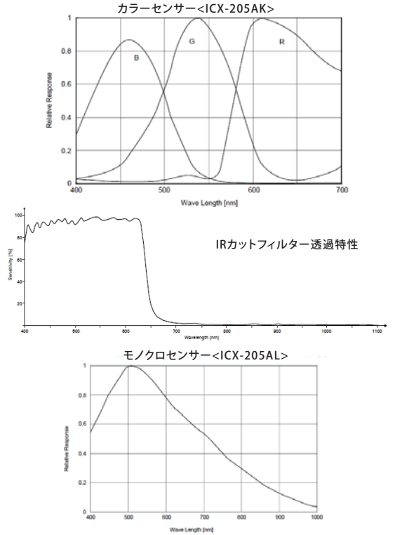
DFK41AU02/DFK41BU02/DMK41AU02/DMK41BU02では、CCDセンサーにSony製ICX-205Aを搭載しています。カラーカメラにはIRカットガラスがカメラケースに固定されており、モノクロカメラには何もついていません。
